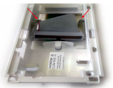
Bild 3 Verlängerungskabel anschließen (BM wird später gesteckt)
